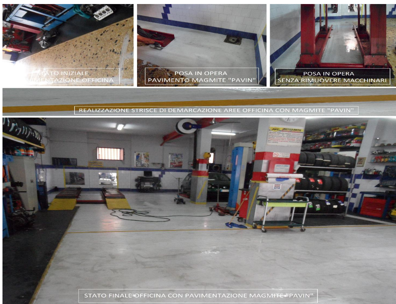
Fig. 4: FOTO IN ALTO: a) visione del pavimento ante opera; b) e c) particolari in fase esecutiva; FOTO IN BASSO: visione post opera "MAGMITE PAVIN".
